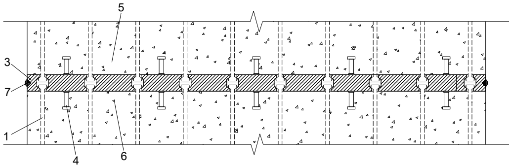
(a) 预应力钢棒焊接连接接头
