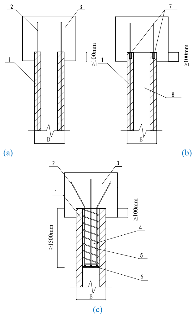
图 5-7 预制墙板与压顶梁连接构造
