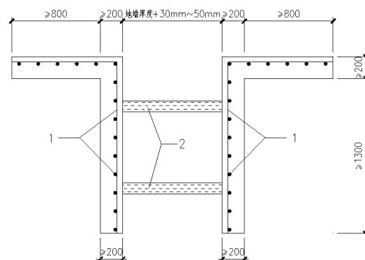
(a)倒“L”型导墙示意图
