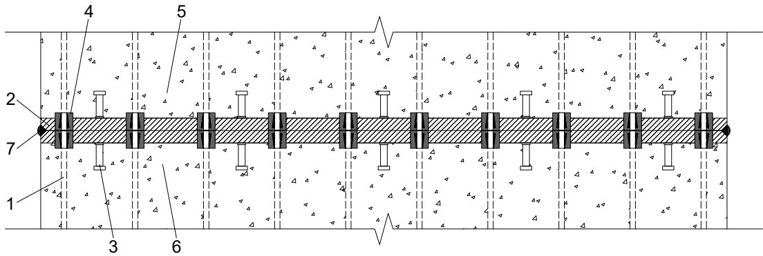
图 5.4.4 预制墙板焊接连接示意图
