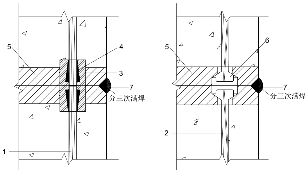
(a) 高强钢绞线焊接连接接头构造
