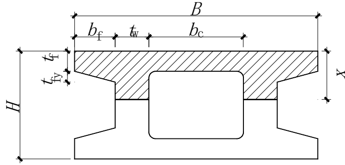
图 4.3.3-3 混凝土受压区高度小于翼缘厚度
