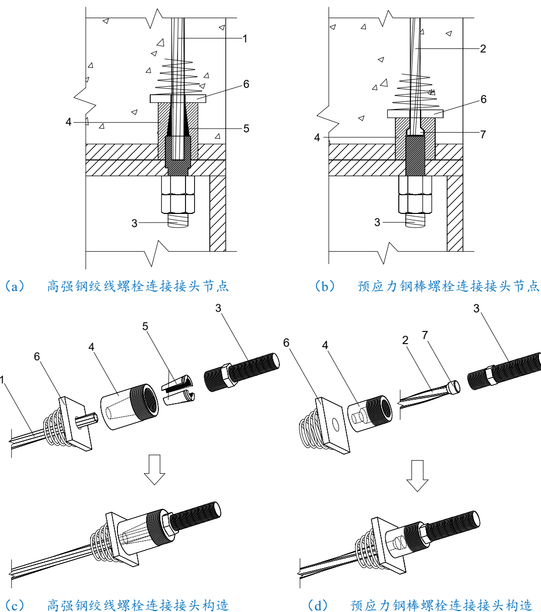
图 5-6 预应力筋螺栓连接接头
