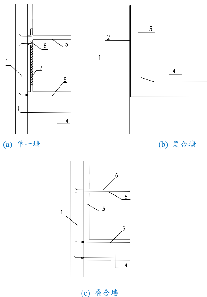
图 5-8 装配式地下连续墙二墙合一的应用形式
