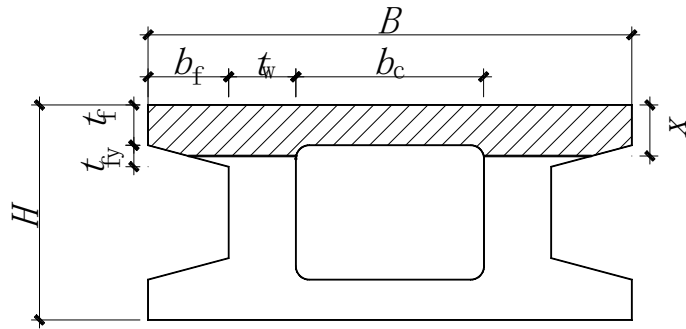
图 4.3.3-2 混凝土受压区高度小于翼缘厚度
