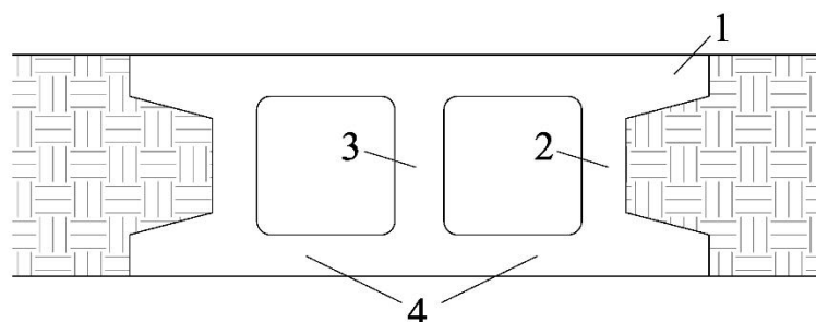
图 4-2 预制墙板局部位置示意
