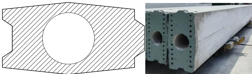
(b) 离心成型凹凸榫墙板
