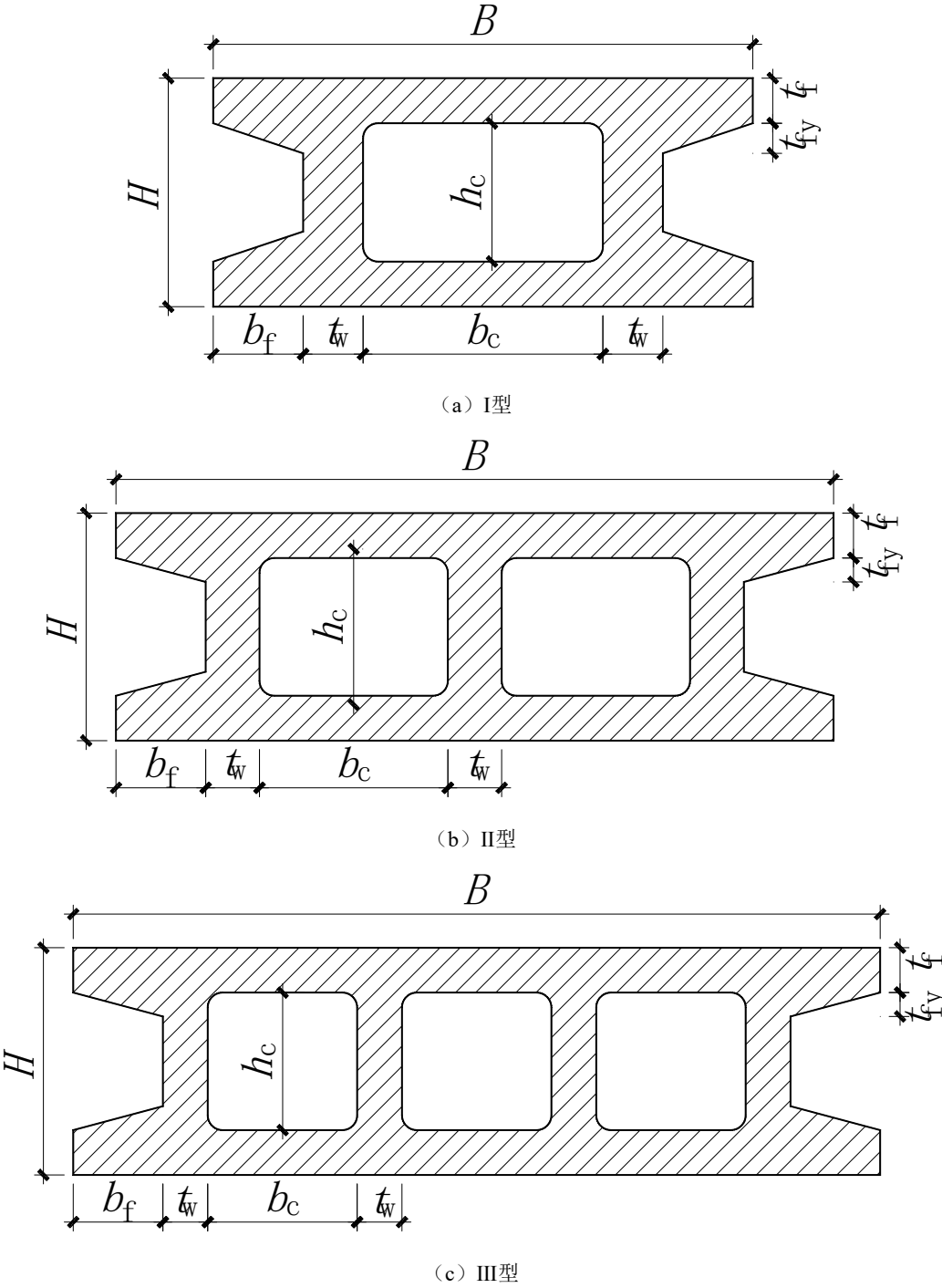
图 A.0.1-1 两侧凹榫型预制墙板截面形式示意图
