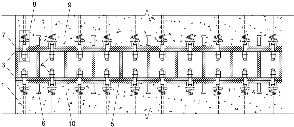
(a) 预应力钢棒螺栓连接接头
