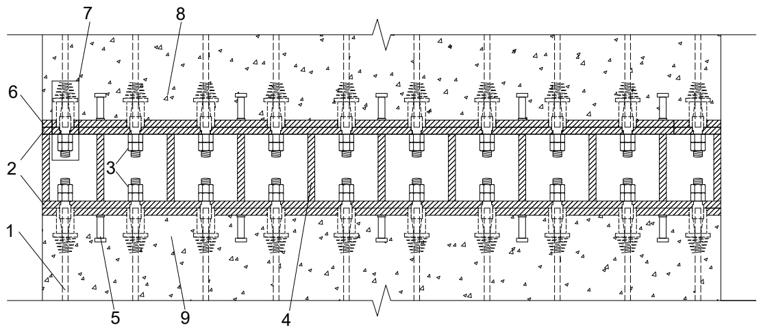
(a) 上下节预制墙板连接示意
