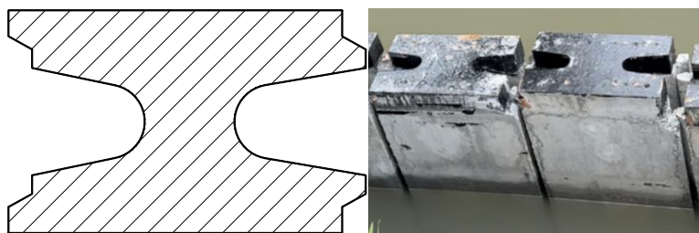
(c) 宽翼缘H型墙板
