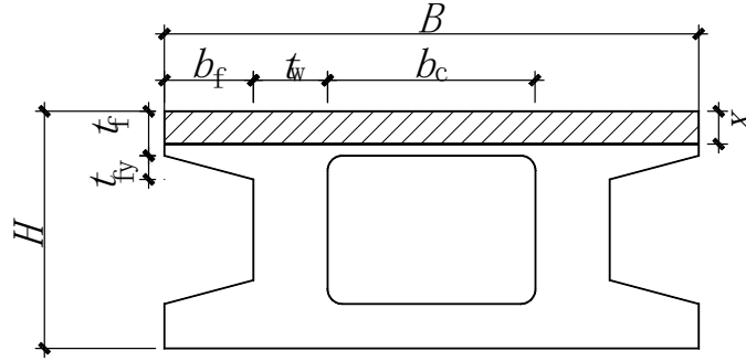
图 4.3.3-1 混凝土受压区高度小于翼缘厚度
