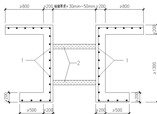
(b)“[”型导墙示意图
