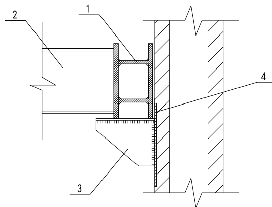
图 5-6 预制墙板与钢腰梁连接构造
