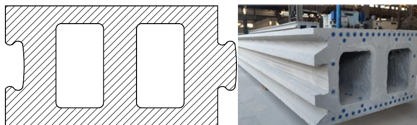
(a) 浇筑成型凹凸榫墙板
