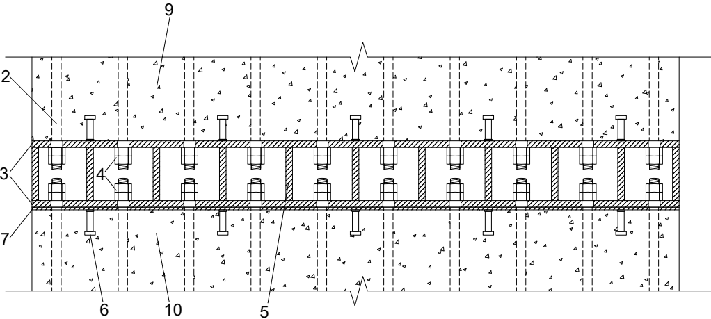
(b) 非预应力筋螺栓连接接头
