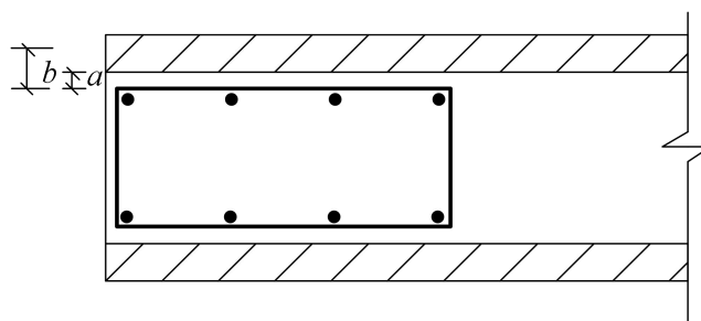
图6.4.13 边缘构件区域墙模保护层厚度示意图
