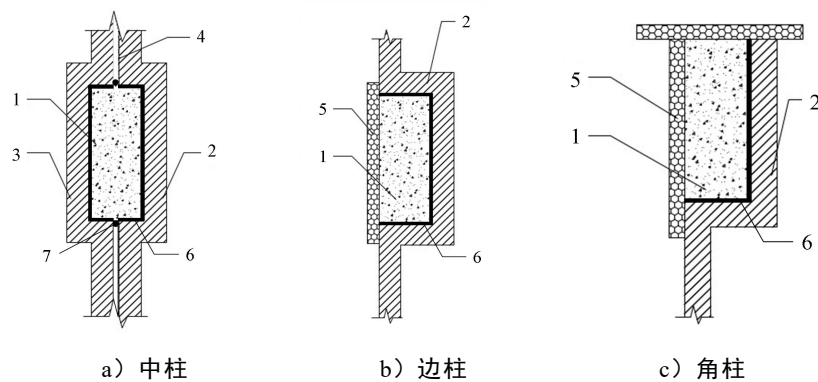
图6.2.16 箱模式模块与现浇混凝土柱的水平布置示意
