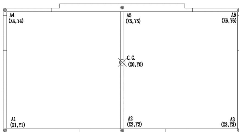
图11 模块吊点布置示意图
