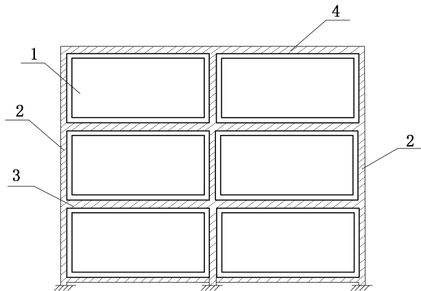
图6.2.14 模块化现浇结构示意图
