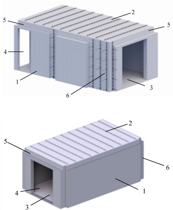
图2 箱模式模块
