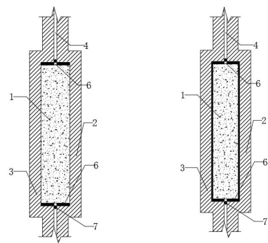
a) 端部设置隔断 b) 长、短边均设置隔断 图7 箱模式模块与现浇剪力墙的水平布置示意
