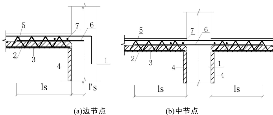
图6.2.20 无外伸纵筋的板端支座构造示意
