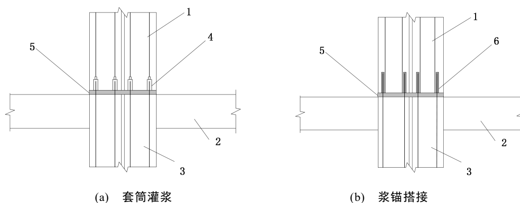
图 6.2.5 堆叠框架结构连接节点构造
