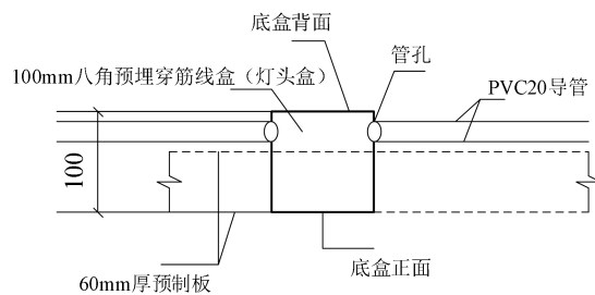
图13 100 mm深灯头盒吸顶安装大样图
