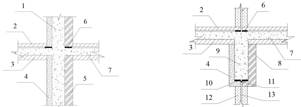
(a) 叠合剪力墙式模块与剪力墙、楼板连接节点 (b) 叠合剪力墙式模块与梁、楼板连接节点
