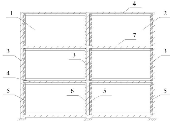
图 6.2.8 模块化叠合剪力墙结构示意图
