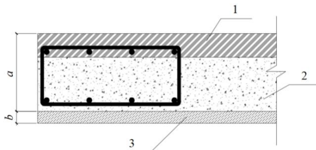
图6.4.12 边缘构件区域叠合剪力墙计算厚度示意图
