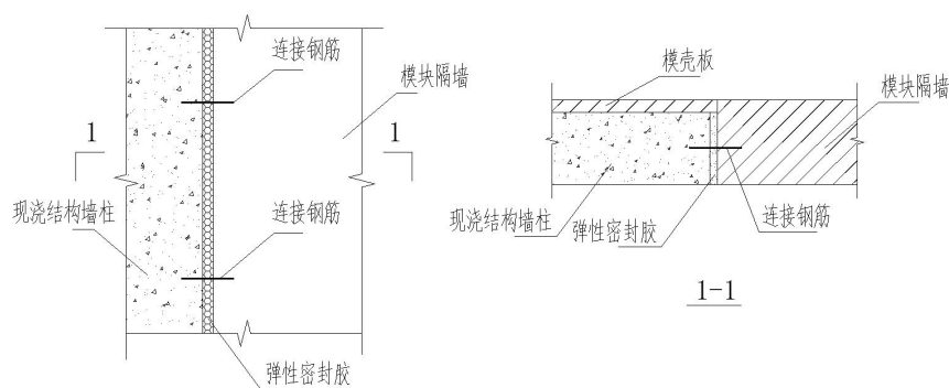
图6 模块单元外墙与现浇竖向结构构件连接节点示意
