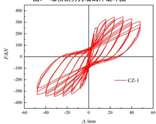
图10 墙模剪力墙滞回曲线
