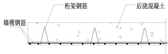
图8 墙模钢筋构造示意图
