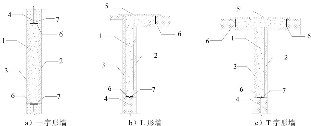
图6.2.17 箱模式模块与现浇剪力墙的水平布置示意
