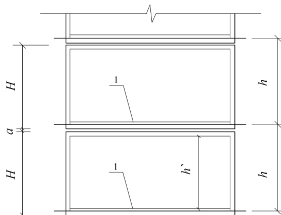
图5.2.5-1 堆叠框架结构竖向布置及建筑层高
