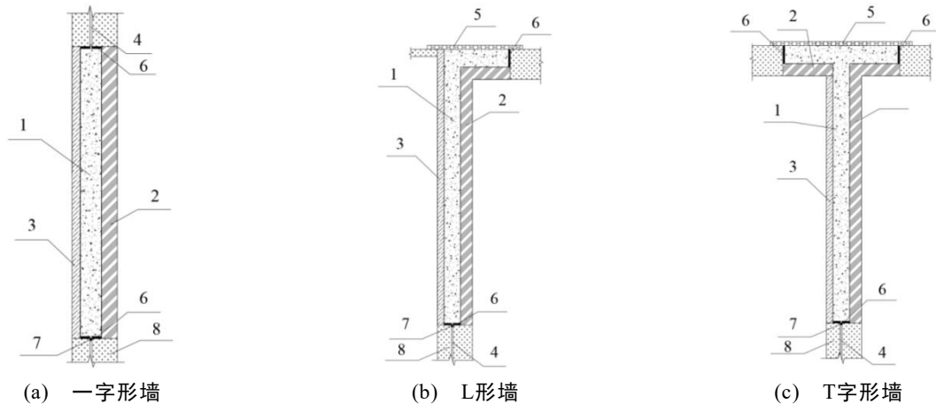
图 6.2.12 构造边缘构件叠合剪力墙式模块与后浇部分的水平布置示意
