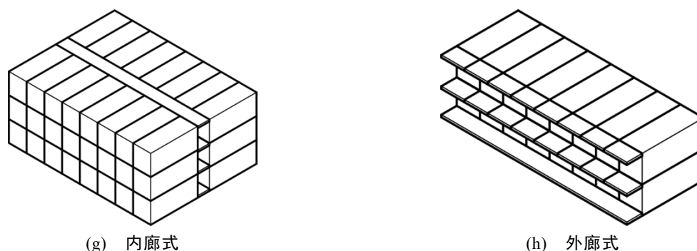
图5.3.4 框架式模块单元组合形式示意图
