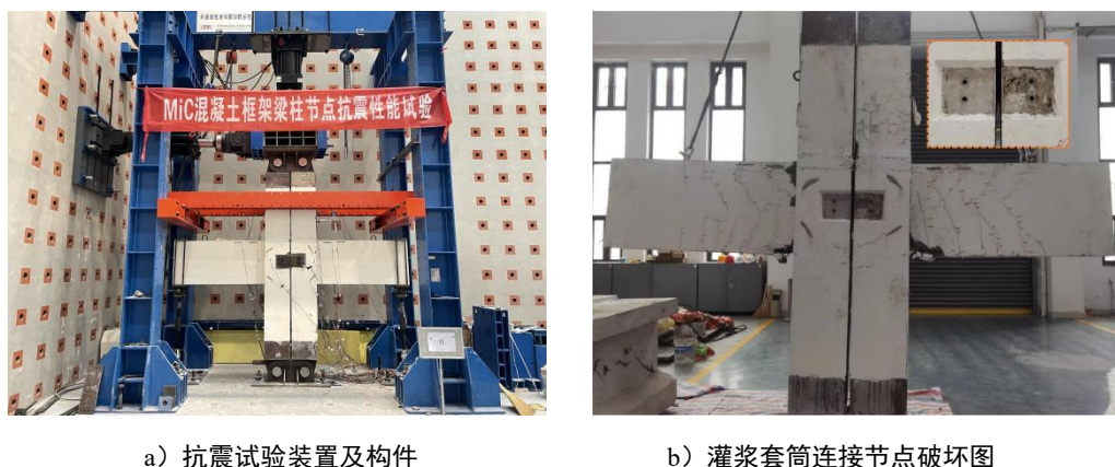
图4 框架式模块连接节点抗震性能试验
